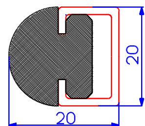
Geländerführung
