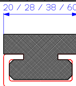
Gleitflachprofil
