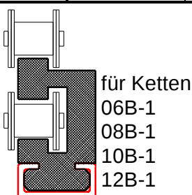
Etagenprofil
