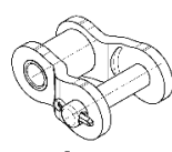
gekröpftes Glied mit Splint
