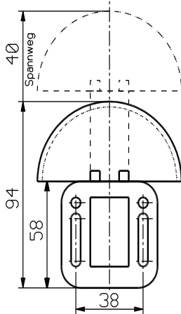
Größe 0 (1-Feder-System, Kunststoffgehäuse)
