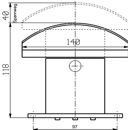
Größe 1 (3-Feder-System, Stahlgehäuse)
