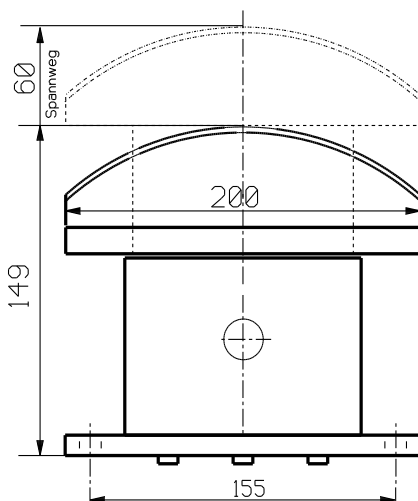
Größe 2 (3-Feder-System, Stahlgehäuse)
