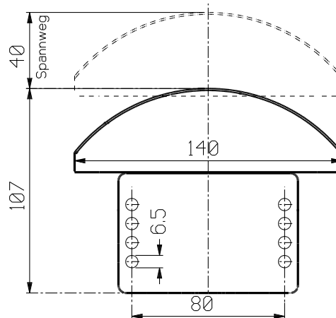
Größe 30 (3-Feder-System, Kunststoff)
